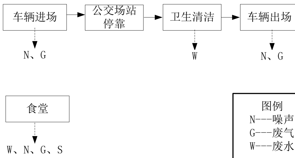
图 3 运营期产污工艺流程图
