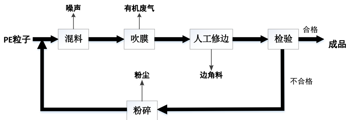
图 5-1 项目薄膜袋工艺流程图
