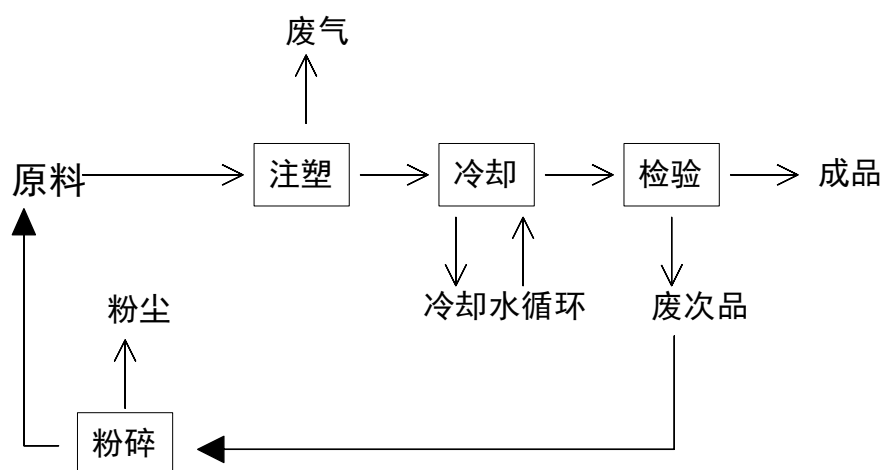
图 1-3 项目薄膜袋工艺流程图
