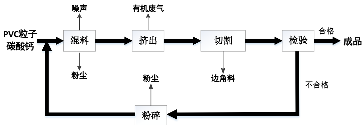
图 5-2 项目塑料管工艺流程图
