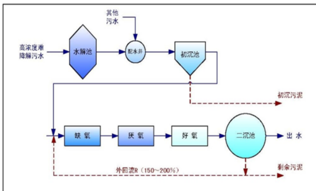
图 2-2 钱江污水处理厂二期工程（12 万 m 3 /d）处理工艺流程图
